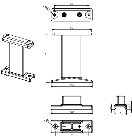
Führungsschienenhalter VL Av (2-01410-PU11X)
