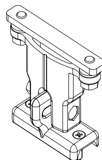
Halter der Führungsleiste Standard SA
