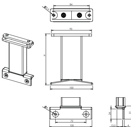
Führungsschienenhalter VL Bv (2-01411-PU11X)
