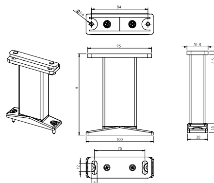
Halter der Führungsleiste Standard SB
