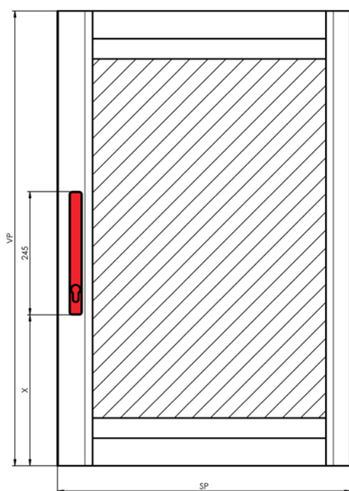
Griff mit Schloss, Betätigung mit einem Schlüssel
