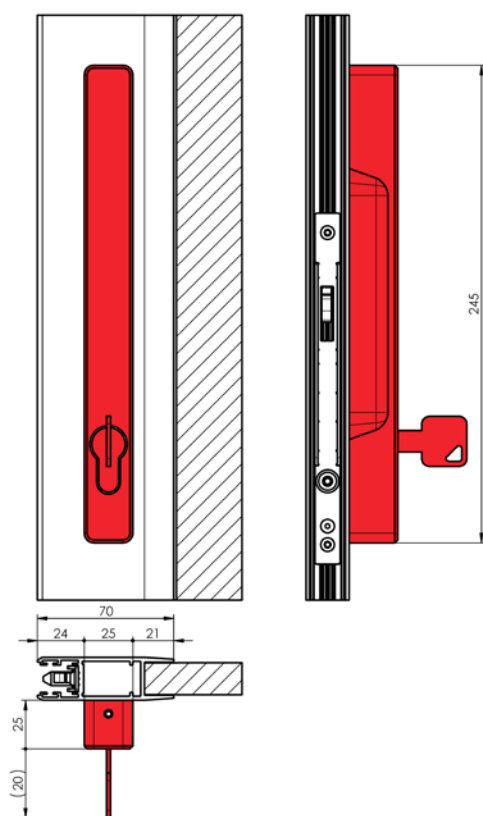
Griff mit Schloss, Betätigung mit einem Schlüssel
