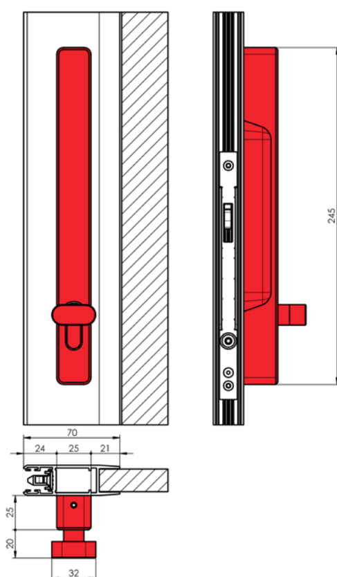
Griff mit Schloss, Betätigung mit einem Knopf
