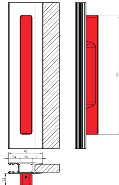
Griff mit Schloss, Betätigung mit einem Knopf
