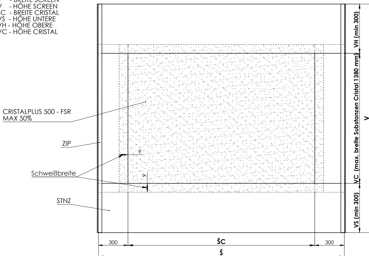
AUSFÜHRUNG DES HORIZONTALSTOFFES CRISTAL FÜR PRODUKTE SCREEN ZIP UND SCREEN ZIP ECONOMY
