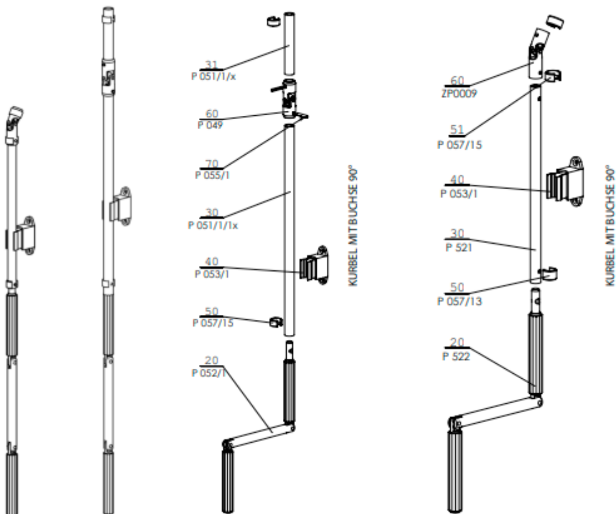
Kurbel für Screen ZIP (2-00868-XXXX-B)
