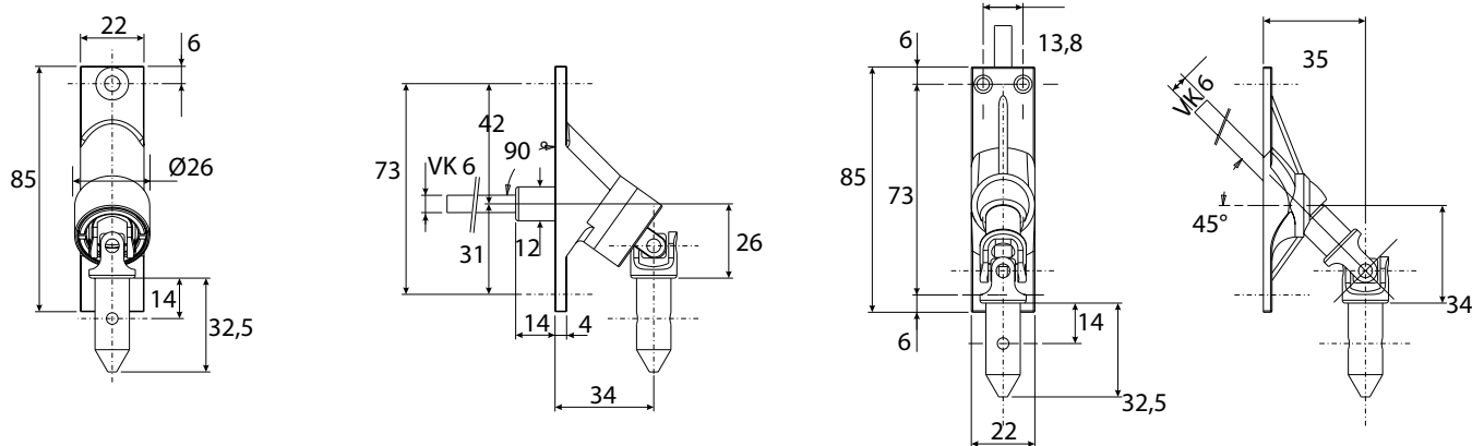
Kardangelenk 90°
