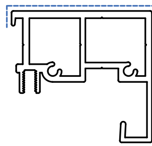
Führungsschiene GS 40 (7-303770-0000)
