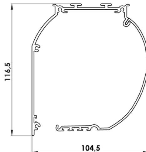
Oberprofil CT 105
