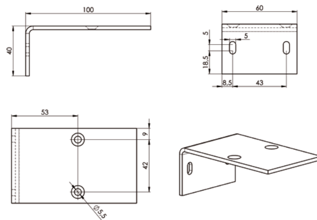
Führungsschiene GS 40 (7-303770-0000)
