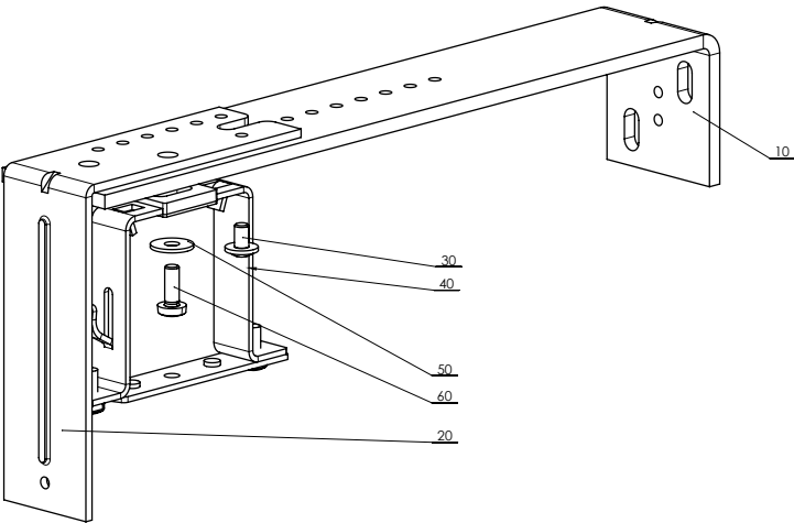
Halter einstellbar – fest 306 – 368 mm P 010/44 (2-01802-0000)
