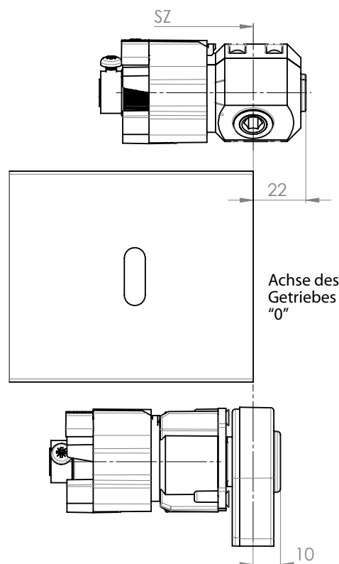
Getriebe Überlappung
