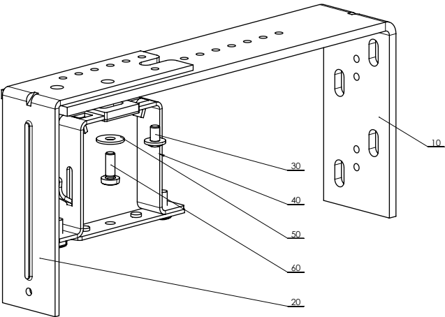
Doppelhalter einstellbar – fest 256 – 318 mm P 010/46 (2-01804-0000)
