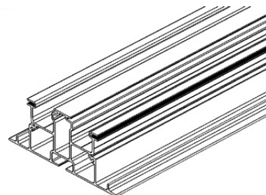
Profil der Führungsleiste, doppelt
