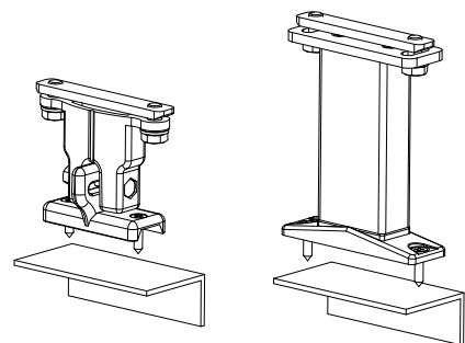
Wandbefestigung
