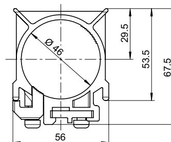
Getriebehalter mit Seilanbindung Geiger, Kunststoff (6-017250)
