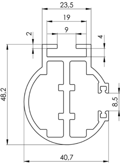
Einseitige Führungsschiene P 018/7 (7-302154)
