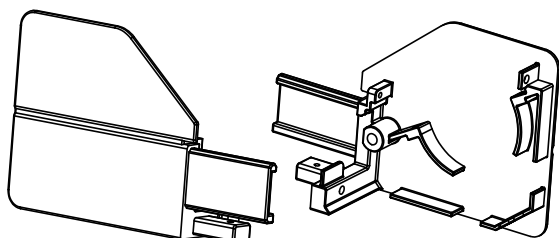
Seitenkonsole LINKS/RECHTS (6-014684 / 6-014685)
